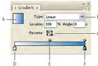
Gradient panel
